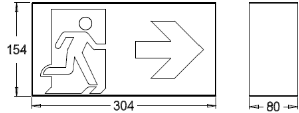
Maßzeichnung (Angaben in mm)
