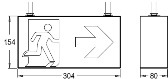
Maßzeichnung (Angaben in mm)
