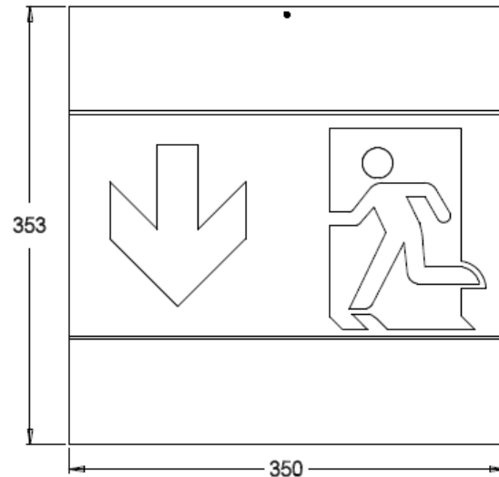
Maßzeichnung (Angaben in mm)
