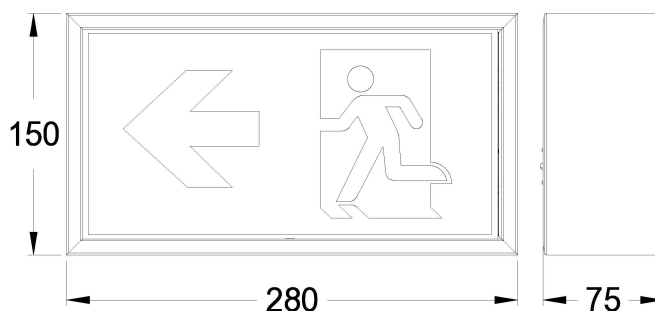
Maßzeichnung (Angaben in mm)
